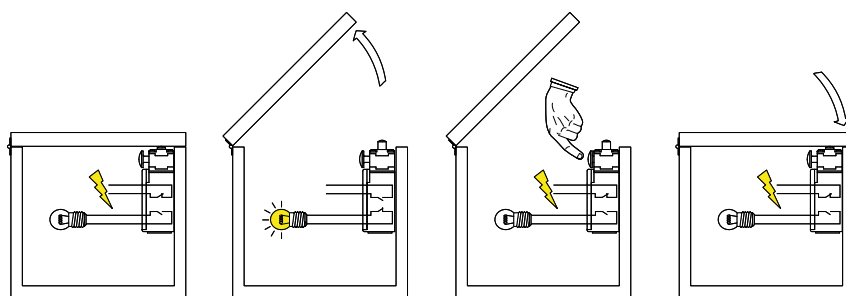
Principio di funzionamento FR 10F1-M2
